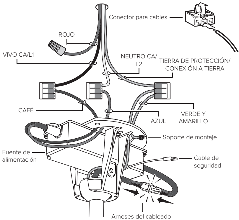
Gráfico de colores de los cables de alimentación
