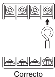
Pelar el cable en el bloque de terminales
