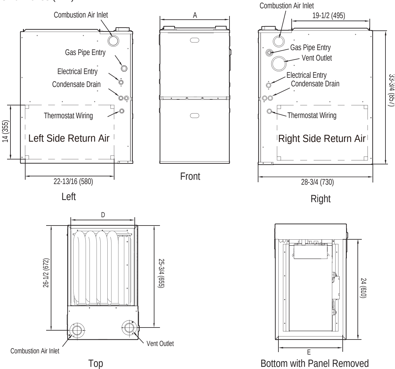
Figure 15: 96 AFUE Gas Furnace Unit Dimensions.
