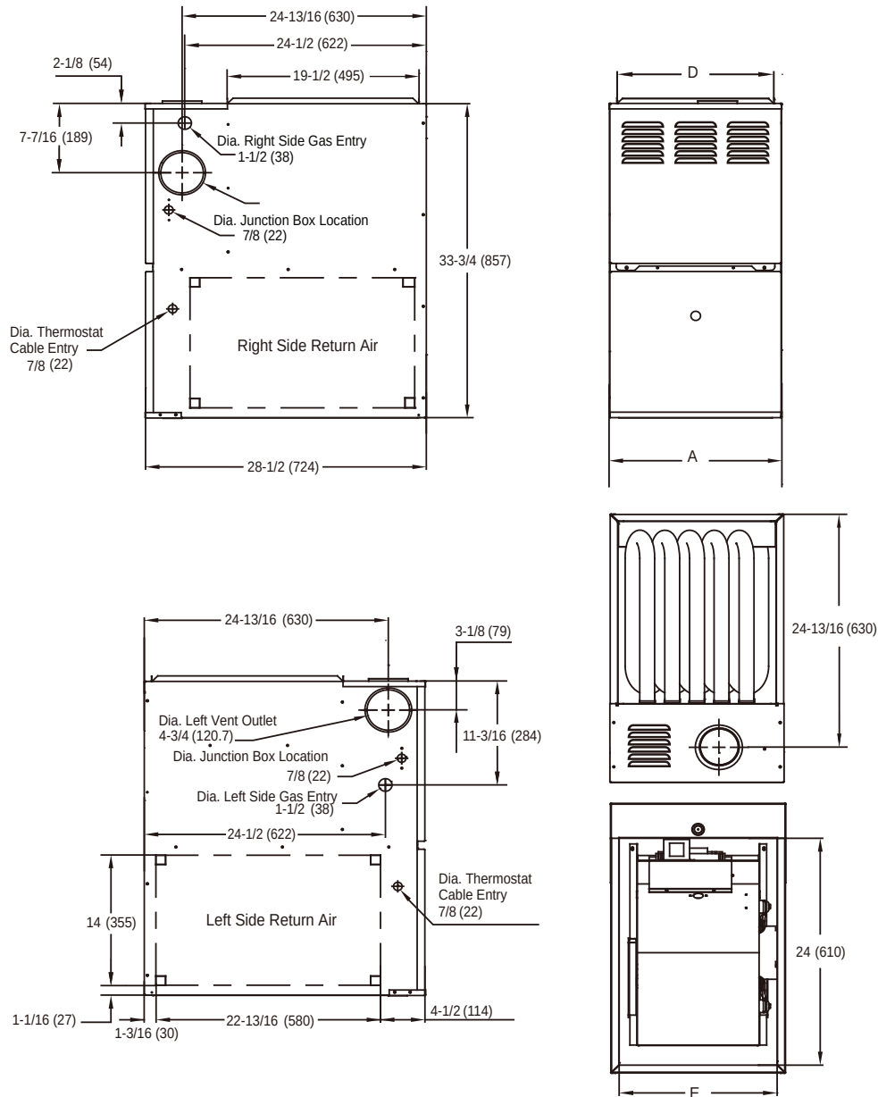
Figure 14: 80 AFUE Gas Furnace Unit Dimensions.
