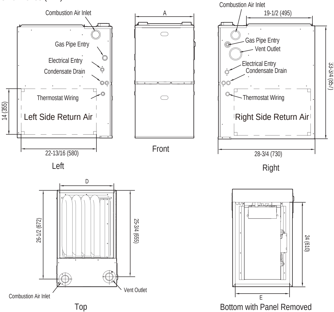
Figure 16: 96 AFUE Gas Furnace Unit Dimensions.
