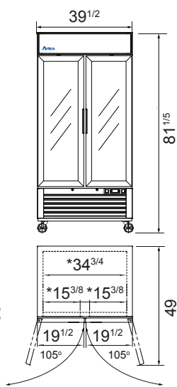
MCF8732GR
