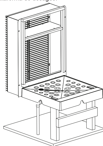
Conexión de la tubería de desagüe sobre la izquierda de la plataforma
