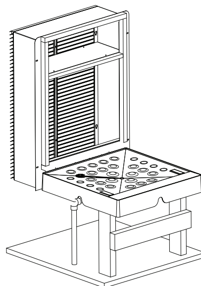
Raccord de la conduite de récupération des fluides à gauche de la plateforme
