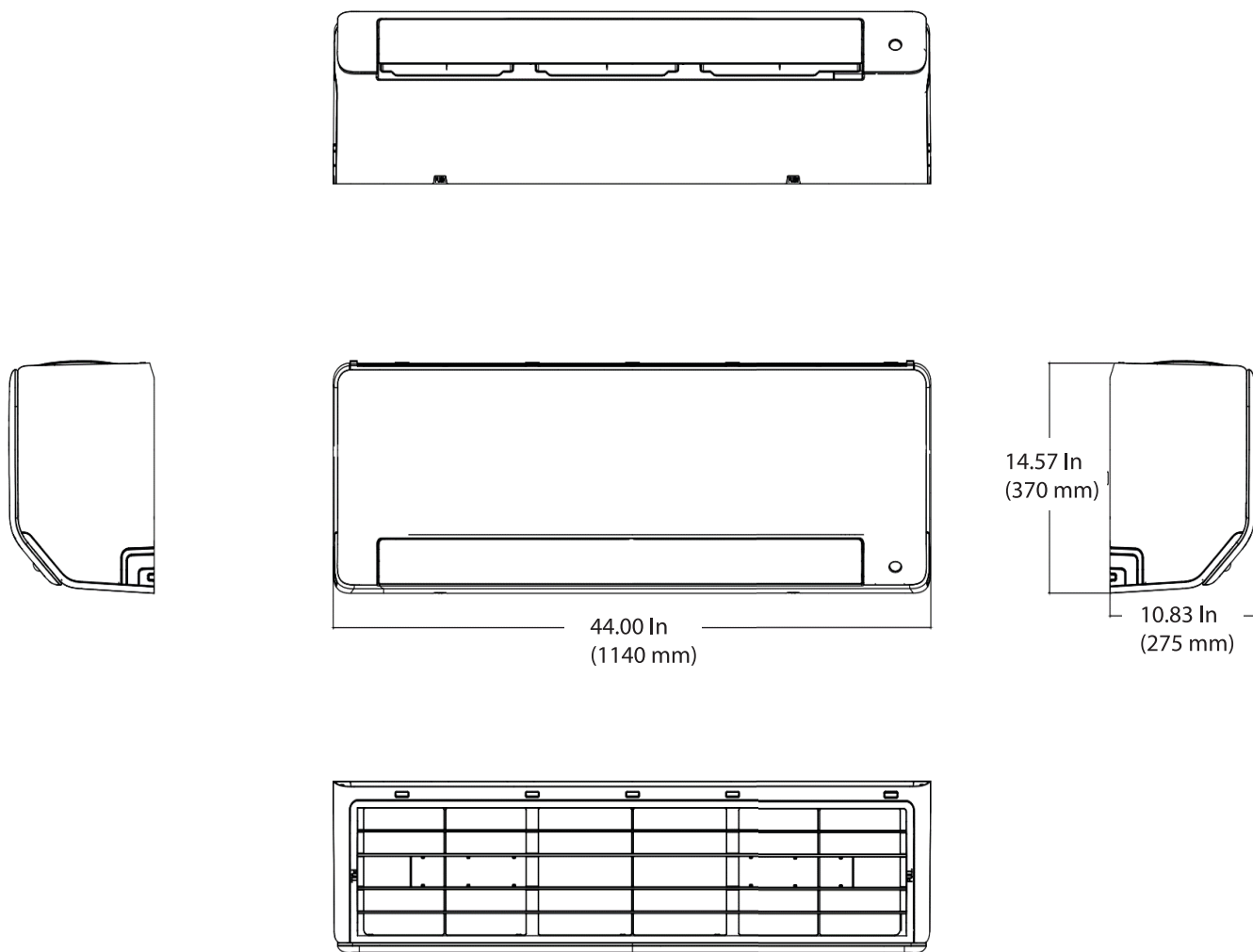
Fig. 4 — Size 18K
